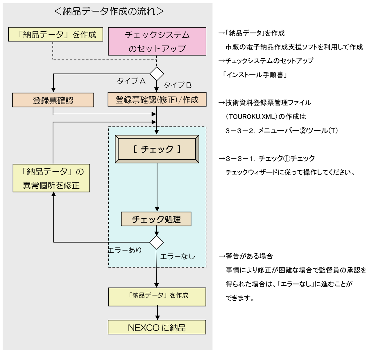
図 3-2 作業の流れ
